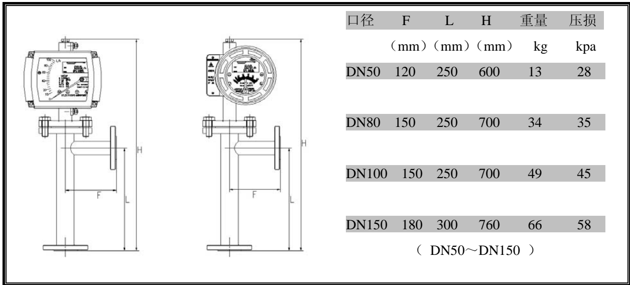
水平安装型：型外形尺寸、重量及压损
