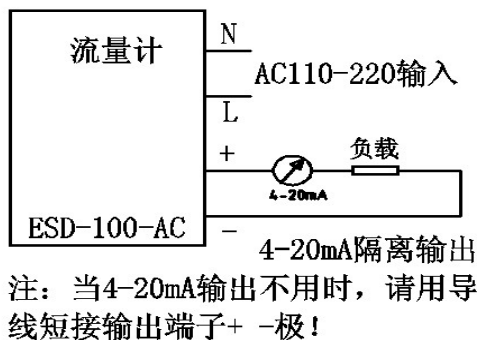
交流供电型接线图
