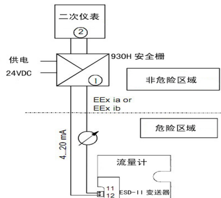
本安系统接线图
