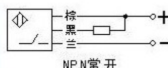
传感器DC三线原理图
