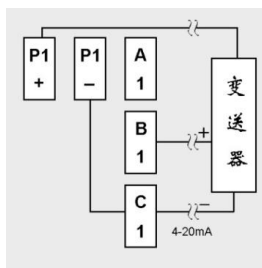
三线制变送器接线图
