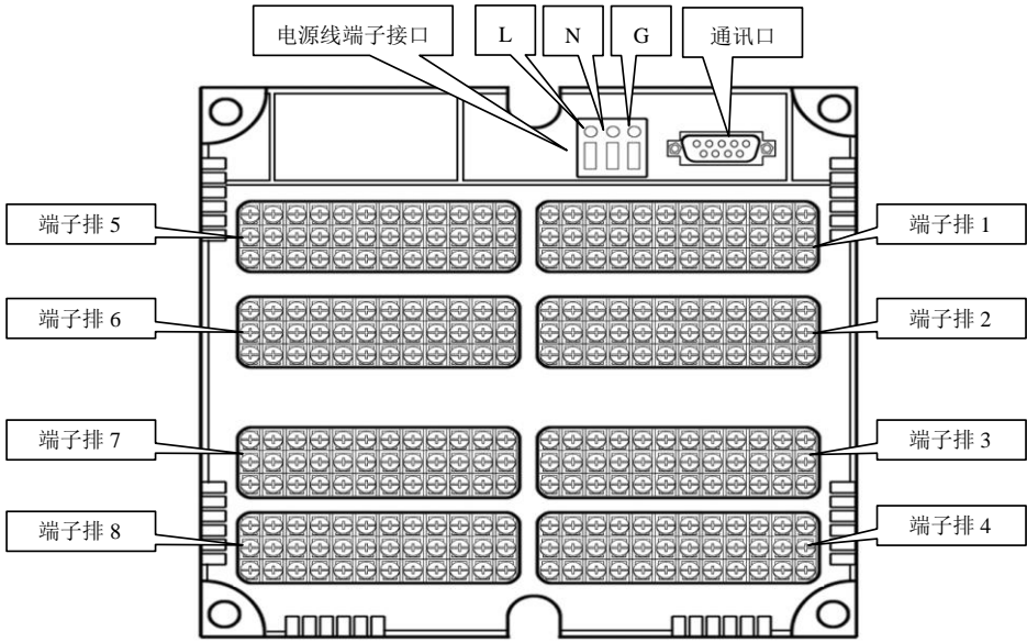
图 2-2-3-A 端子排列图
