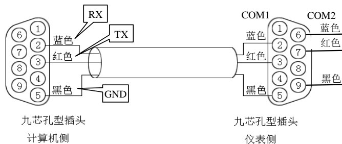
图 2-2-7-A 计算机与仪表间的 RS-232C 通讯线
