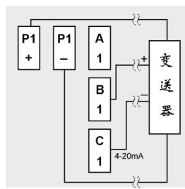
四线制变送器接线图
