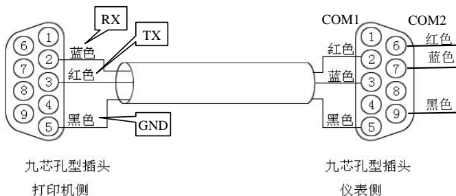
图 2-2-7-B 打印机与仪表间的 RS-232C 通讯线
