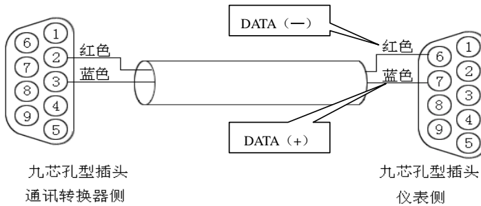
图 2-2-9 通讯转换器与仪表间的 485 通讯线
