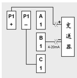
两线制变送器接线图
