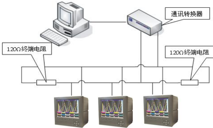
图 2-2-8 485 通讯联网示意图
